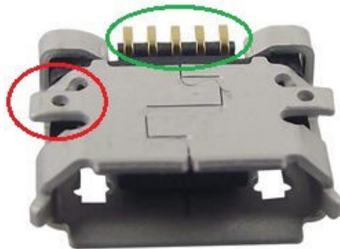
Abbildung 2: USB Buchse
