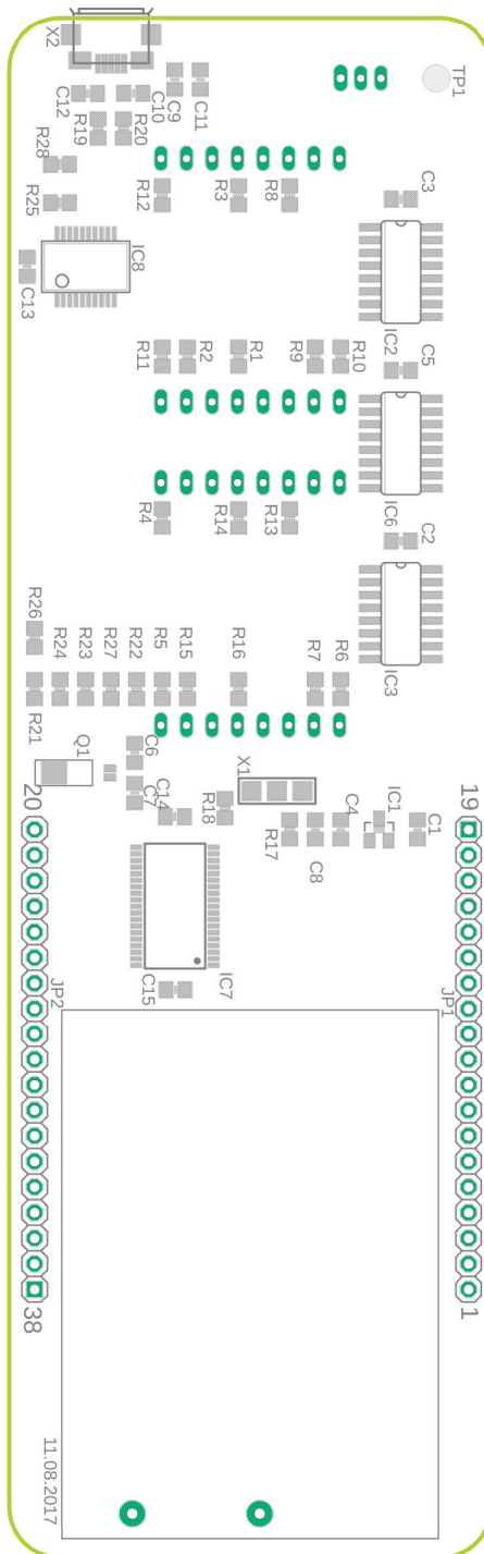
Abbildung 1: Bestückungsplan Unterseite
